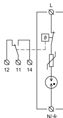
Vnúťorná schéma zapojenia
